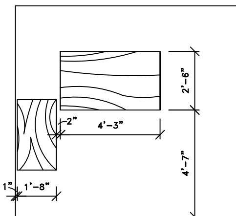
ELEVATION "D" SCALE: 1/4"=1'-0"
