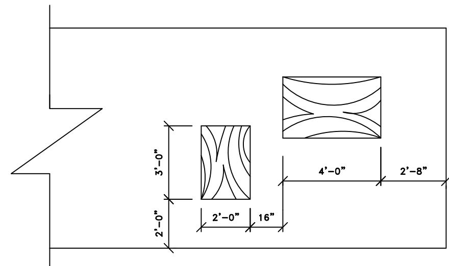
ELEVATION "A" SCALE: 1/4"=1'-0"
