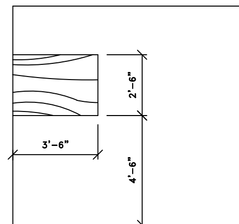
ELEVATION "E" SCALE: 1/4"=1'-0"
