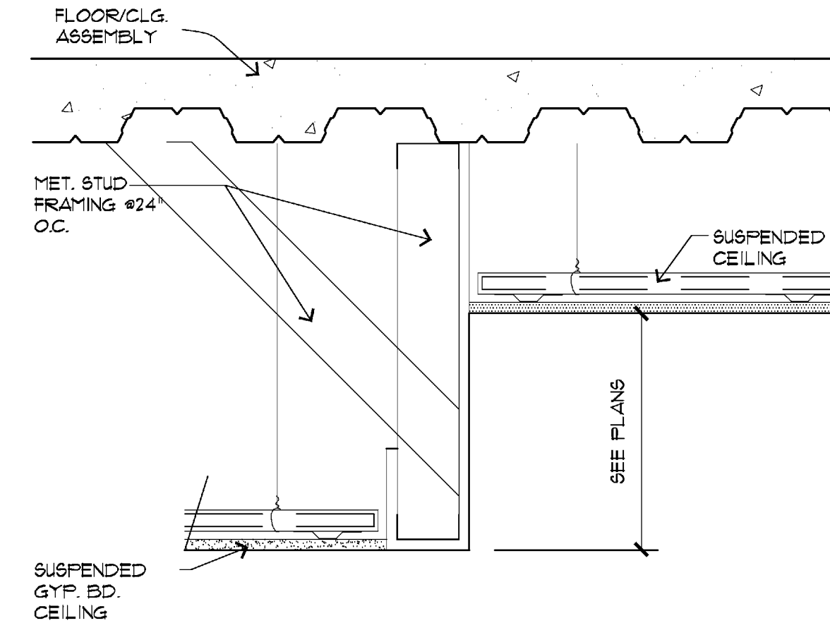
2 CEIL'G DET.(Mtg. Rm.)
