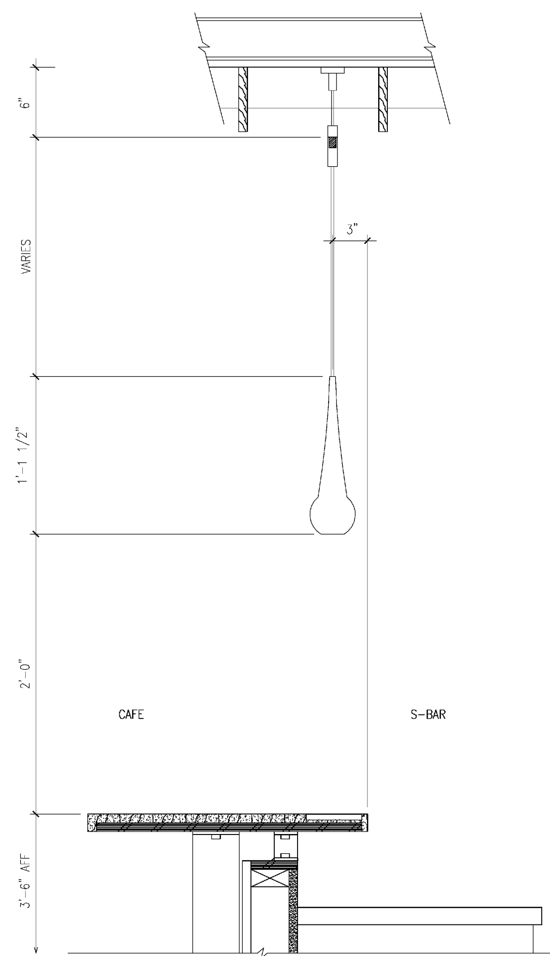
15 PENDANT DETAIL
