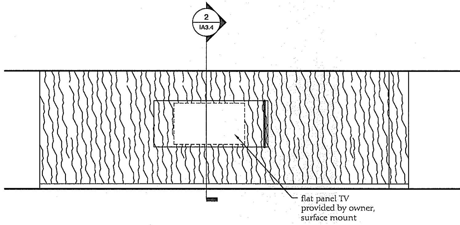
01 Elevation - Upper Lounge T.V.
