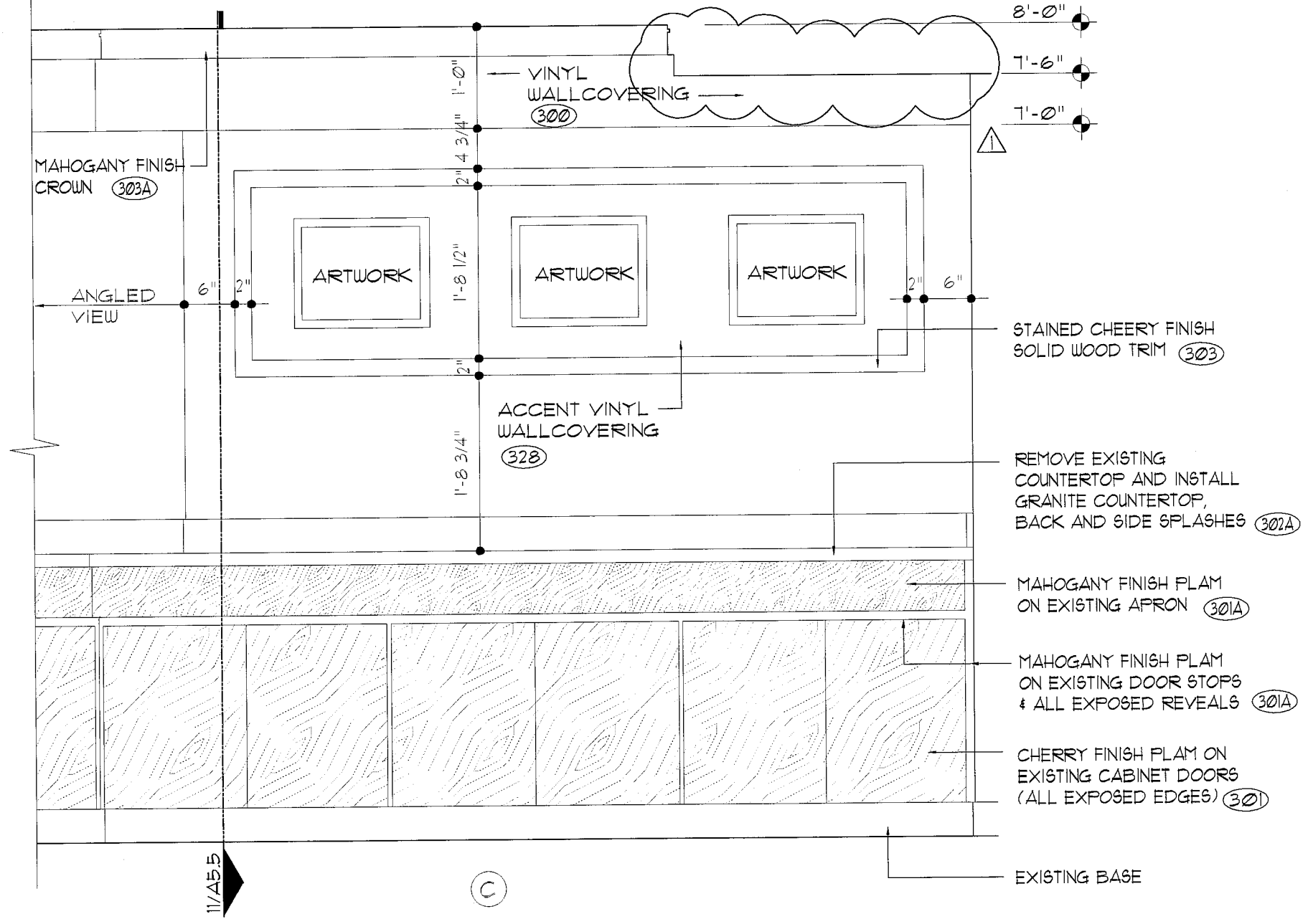
SCALE: 1 1/2" = 1'-0"
