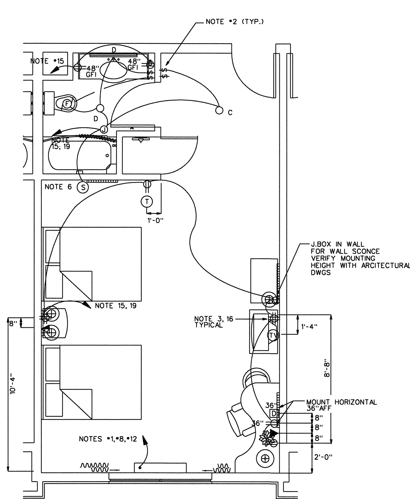
DELUXE DOUBLE QUEEN SCALE: 1/4" = 1'-0"
