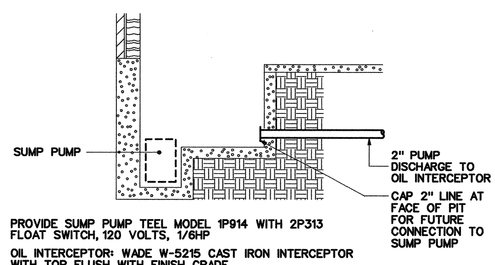
ELEVATOR SUMP DETAIL N.T.S.
