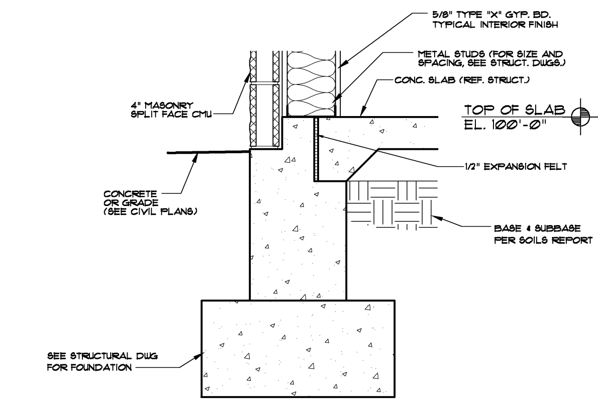
2 SLAB EDGE DETAIL 1" = 1'-0"
