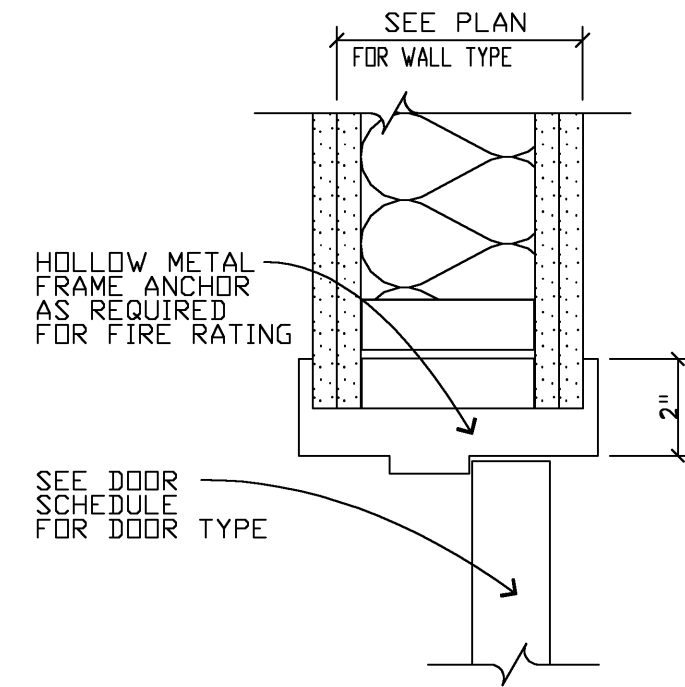
J7 JAMB 3" = 1'-0"
