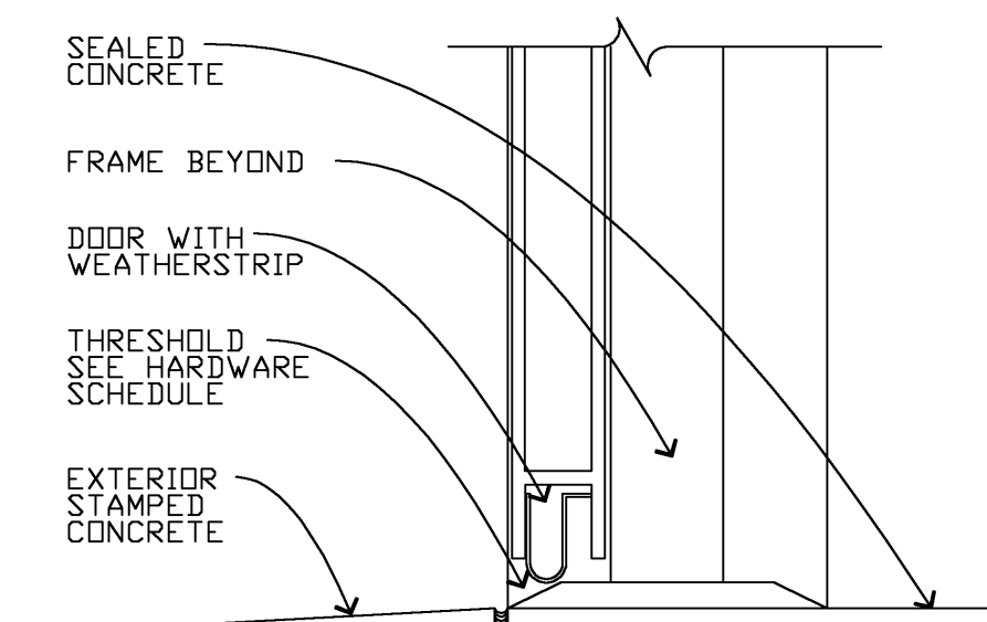
S6 SILL 3" = 1'-0"
