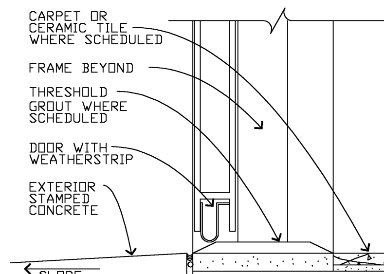
S4 SILL 3" = 1'-0"
