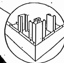
STUD CORNER DETAIL
