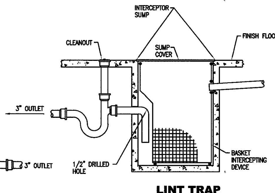
LINT TRAP SCALE: NONE
