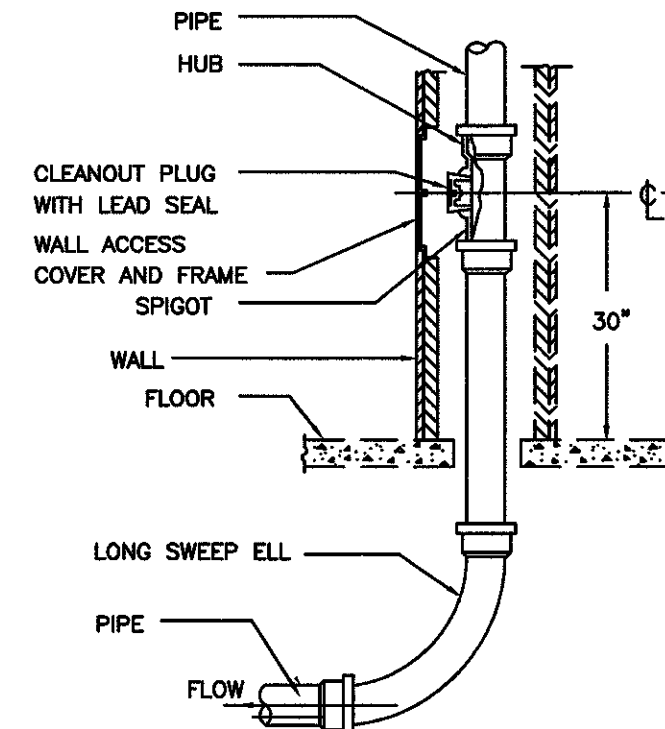
WALL CLEANOUT SCALE: NONE
