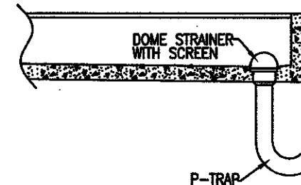
TRENCH DRAIN SCALE: NONE
