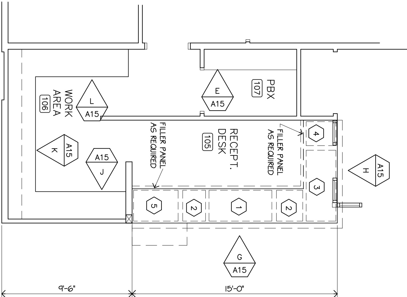
TYP. MODULE LAYOUT
