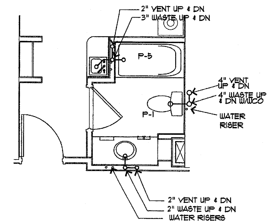
8 TYP. FLR. SUITE 1/4" = 1'-0" AX-X-X
