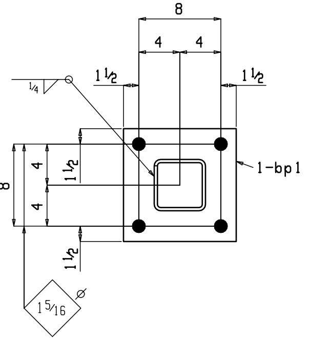
3 COLUMNS 27C1
