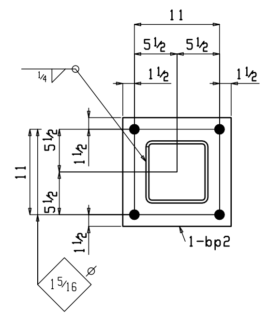
2 COLUMNS 26C2
