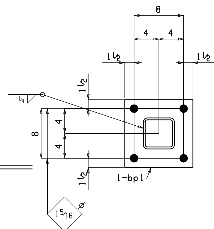
2 COLUMNS 26C1
