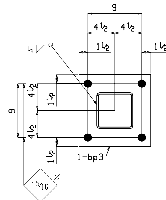
4 COLUMNS 26C3
