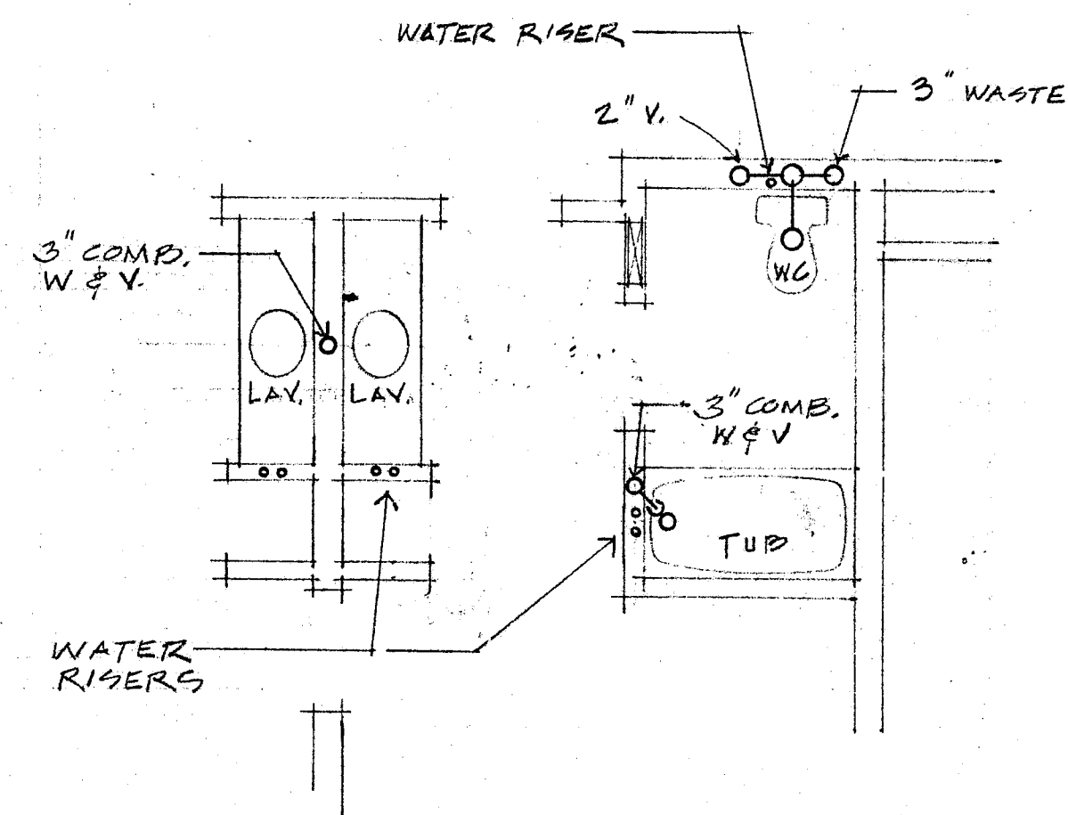
② TYP. FLOOR
